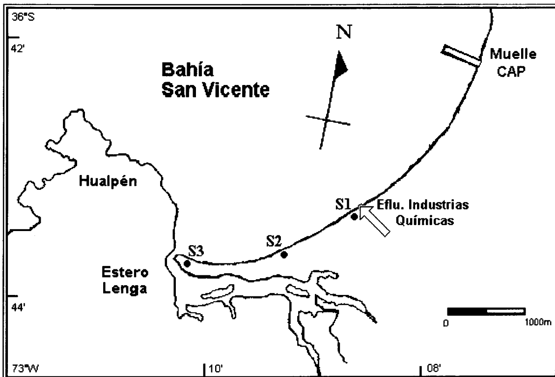
Fig. 1: Localización geográfica de los sitios de estudio (S1, S2 y S3) en playa Lenga, Bahía de San Vicente. La flecha blanca indica la ubicación del punto de evacuación de efluentes de las industrias químicas.
